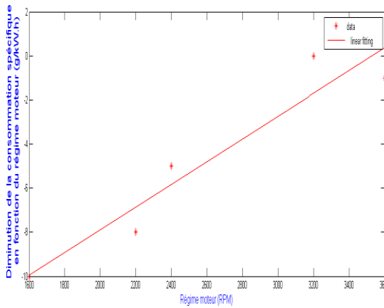
FIGURE 7. L'évolution de la consommation spécifique après la correction de combustion et la pression d'injection
