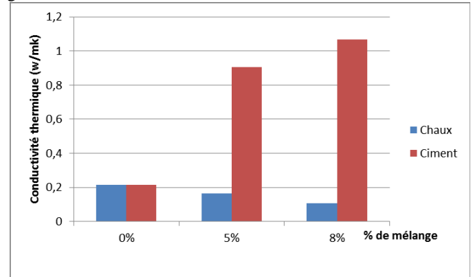
Fig. 2 Influence des ajouts ciment et chaux sur la conductivité thermique du mélange.
