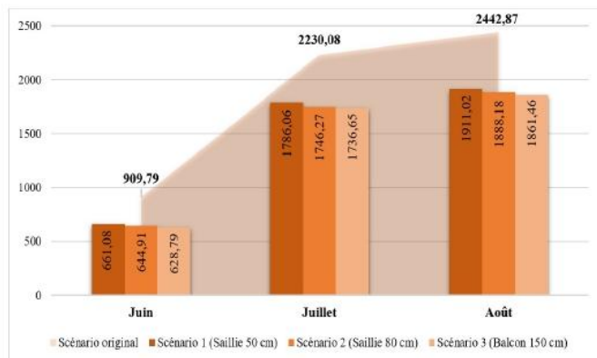
Fig. 3. Consommation d'énergie suite à l'ajout des protections solaires (en kWh)
