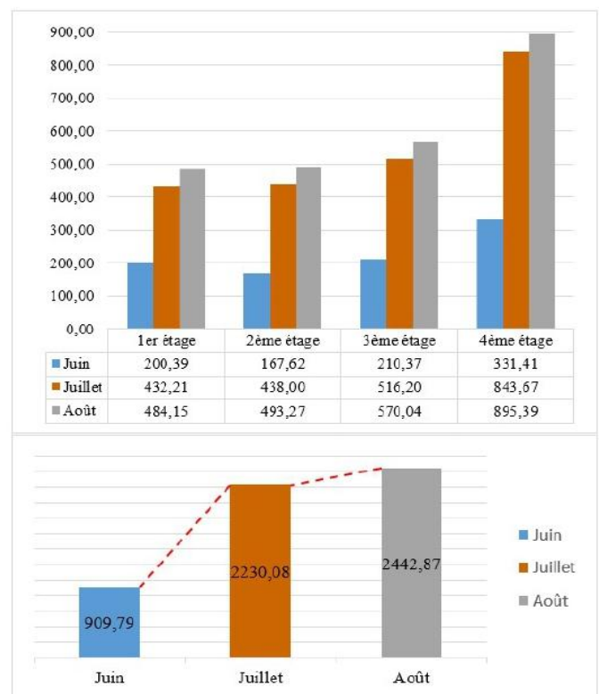
Fig. 2. Les besoins énergétiques de l'immeuble durant la période estivale (en kWh)
