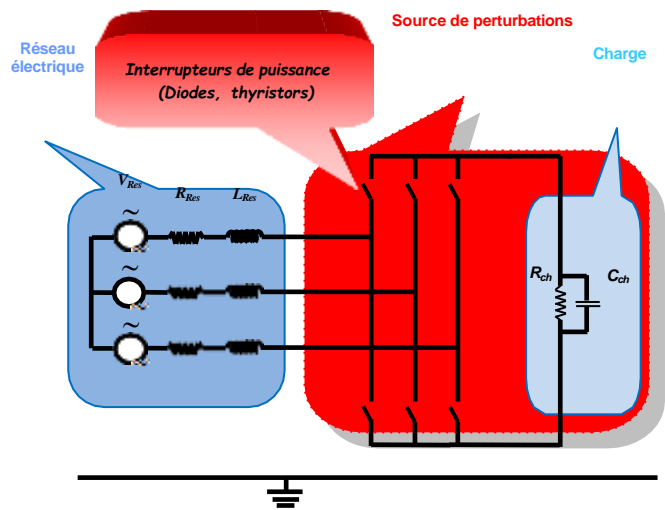
Fig. 1 Structure du pont de diode triphasé débitant sur une charge-Modèle basses fréquences
