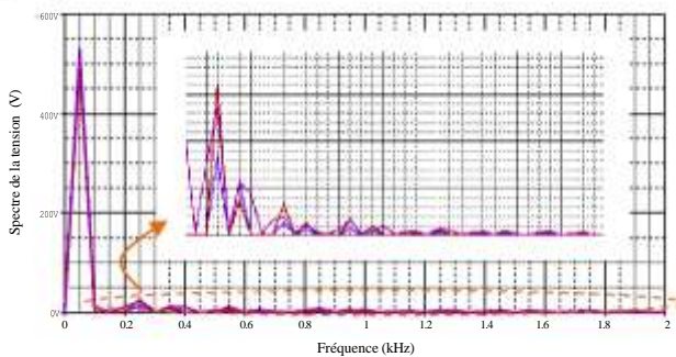
Fig. 4 Spectre fréquentiel de la tension composée à l'entrée du pont redresseur triphasé
