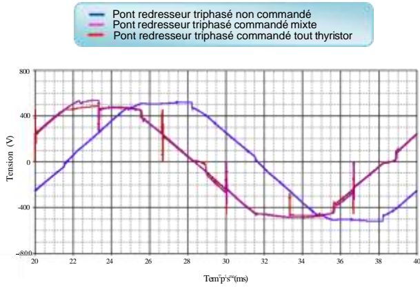
Fig. 2 Variations temporelles de la tension composée à l'entrée du pont redresseur triphasé
