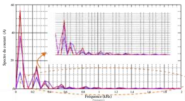
Fig. 5 Spectre fréquentiel du courant de ligne
