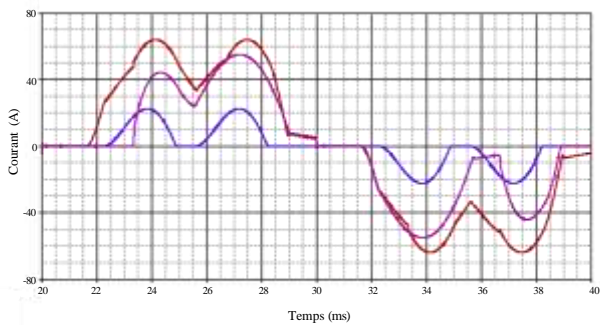
Fig. 3 Variations temporelles du courant de ligne du pont redresseur
