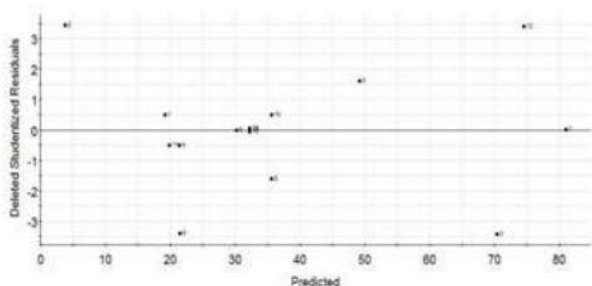
Fig. 3 Tracé des résidus observés en fonction des valeurs prévues.
