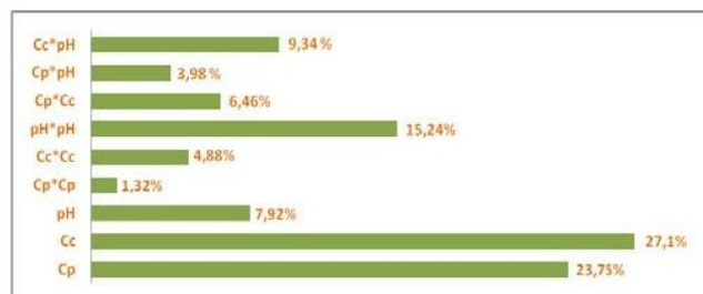
Fig.5 Analyse graphique de Pareto
