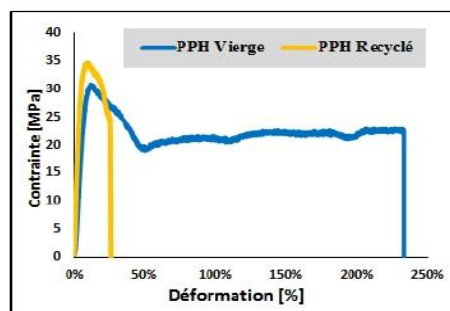
Fig. 2: Courbe contrainte déformation du PP
