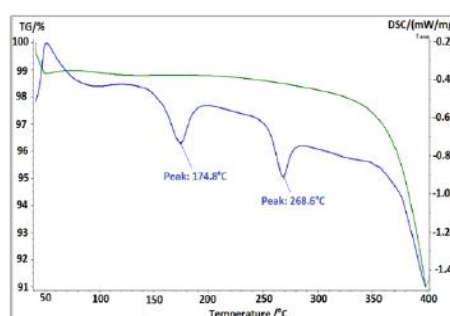
Fig. 4: Analyse par DSC du mélange 50%PPH/50%PA6 recyclé
