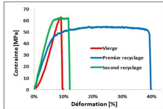
Fig. 4 : Relation Contrainte-Déformation du polymère 100% PA6-6
