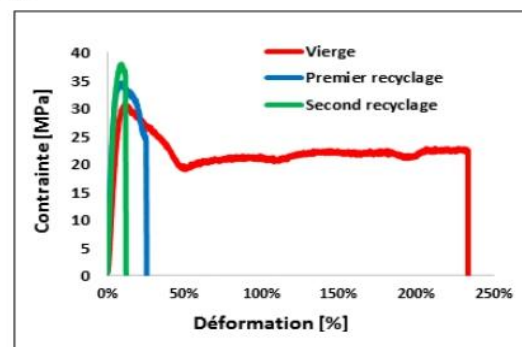
Fig. 5 : Relation Contrainte-Déformation du polymère 100% PPC
