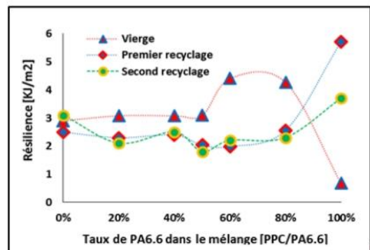
Fig. 10: Variation de la résilience des mélanges vierge et recyclés en fonction du taux de PA dans la matrice PP
