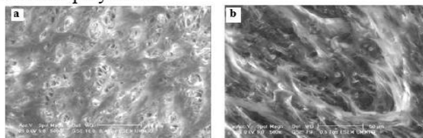
Fig. 4 : Observation au MEB des faciès de rupture du polymère 100%PA vierge et recyclé
