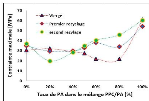
Fig 9 : Variation de la contrainte au seuil d'écoulement des mélanges vierge et recyclés en fonction du taux de PA6.6 dans le mélange PPC/PA6.6
