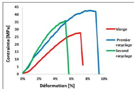
Fig. 6 : Relation Contrainte-Déformation du polymère 50% PPC/50%PA6.6
