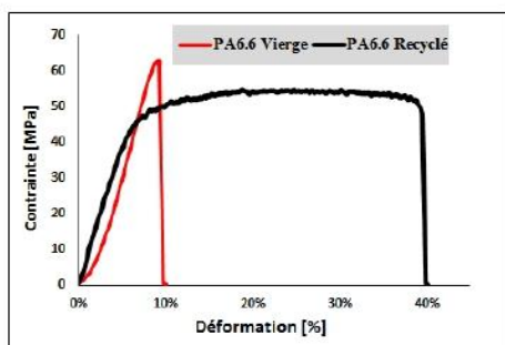
Fig. 1: Courbe contrainte déformation du PA6.6
