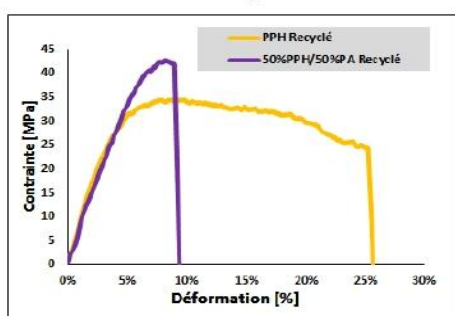
Fig. 3: Courbe contrainte déformation PPH recyclé et du mélange 50%PPH/50%PA6 recyclé
