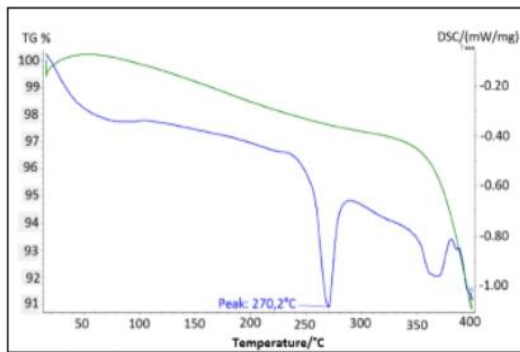
Fig. 2 : Analyse thermique différentielle (DSC) du PPA 6.6
