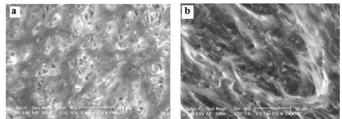
Fig 11 : Observation au MEB des faciès de rupture du polymère 100%PA vierge et recyclé
