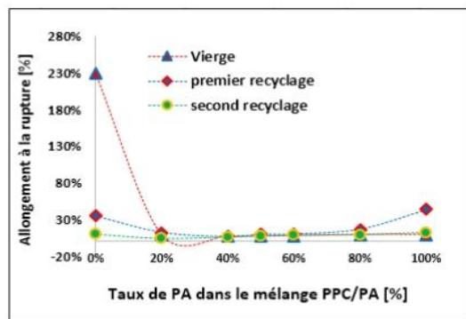
Fig 8 : Variation de l'allongement à la rupture des mélanges vierges et recyclés en fonction du taux de PA dans la matrice PP
