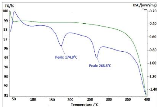
Fig. 3 : Analyse thermique différentielle (DSC) du 50%PPC/50%PA6.6
