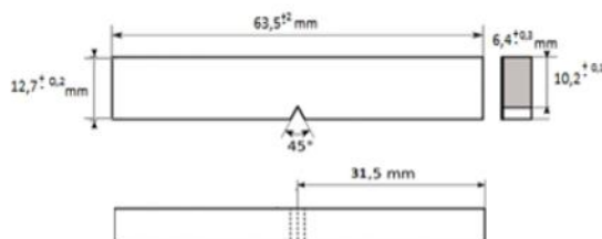
Schéma 2 Géométrie des éprouvettes de résilience
