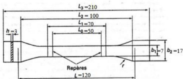
Schéma 1 Géométrie des éprouvettes de traction conforme à la norme NF EN ISO 527-2
