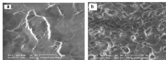
Fig. 12 : Observation au MEB des faciès de rupture du polymère 100%PP vierge et recyclé
