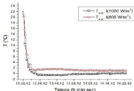
Fig. 8 Changement de la température d'évaporation pendant le temps dans l'évaporateur.
