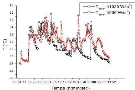
Fig. 7 Développement de la température de condensation dans le condenseur pour l'irradiation 1020 \text{ W/m}^2 et 800 \text{ W/m}^2 .
