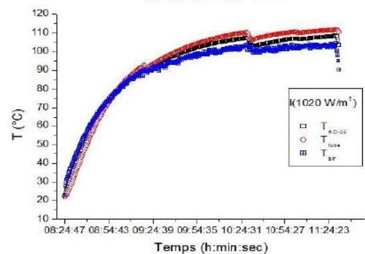
Fig. 5 Distribution de la température dans le générateur tubulaire pour l'irradiation 1020 W/m 2 .
