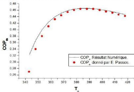
Fig. 2 Les valeurs du COP th par rapport à la variation de la température de régénération T g . (T a =25 °C, T c =30 °C, T e =-5 °C)
