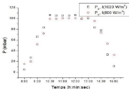
Fig. 6 Variation temporelle de la pression dans le générateur tubulaire.
