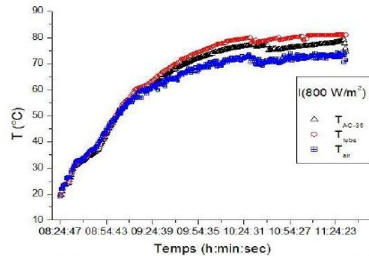
Fig. 4 Distribution de la température dans le générateur tubulaire pour l'irradiation 800 W/m 2 .
