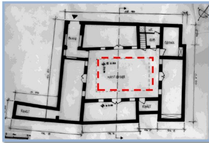
Plan. N°01 : RDC de l'organisation des espaces autour du patio. Dar Seladji quartier R'hib, Tlemcen.
