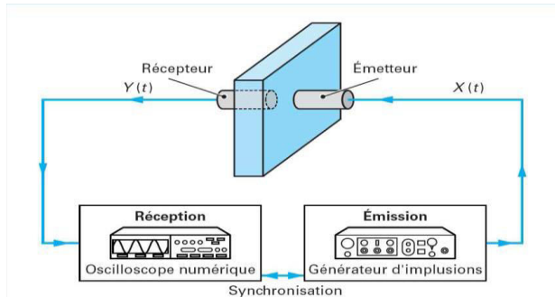
Figure 2 : Schéma descriptif de transmission en contact direct [13]
