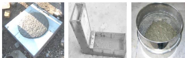
Figure 1 : Essais pour la caractérisation du béton testé à l'état frais
