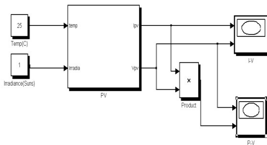
Fig. 3 Model Simulink de la cellule PV
